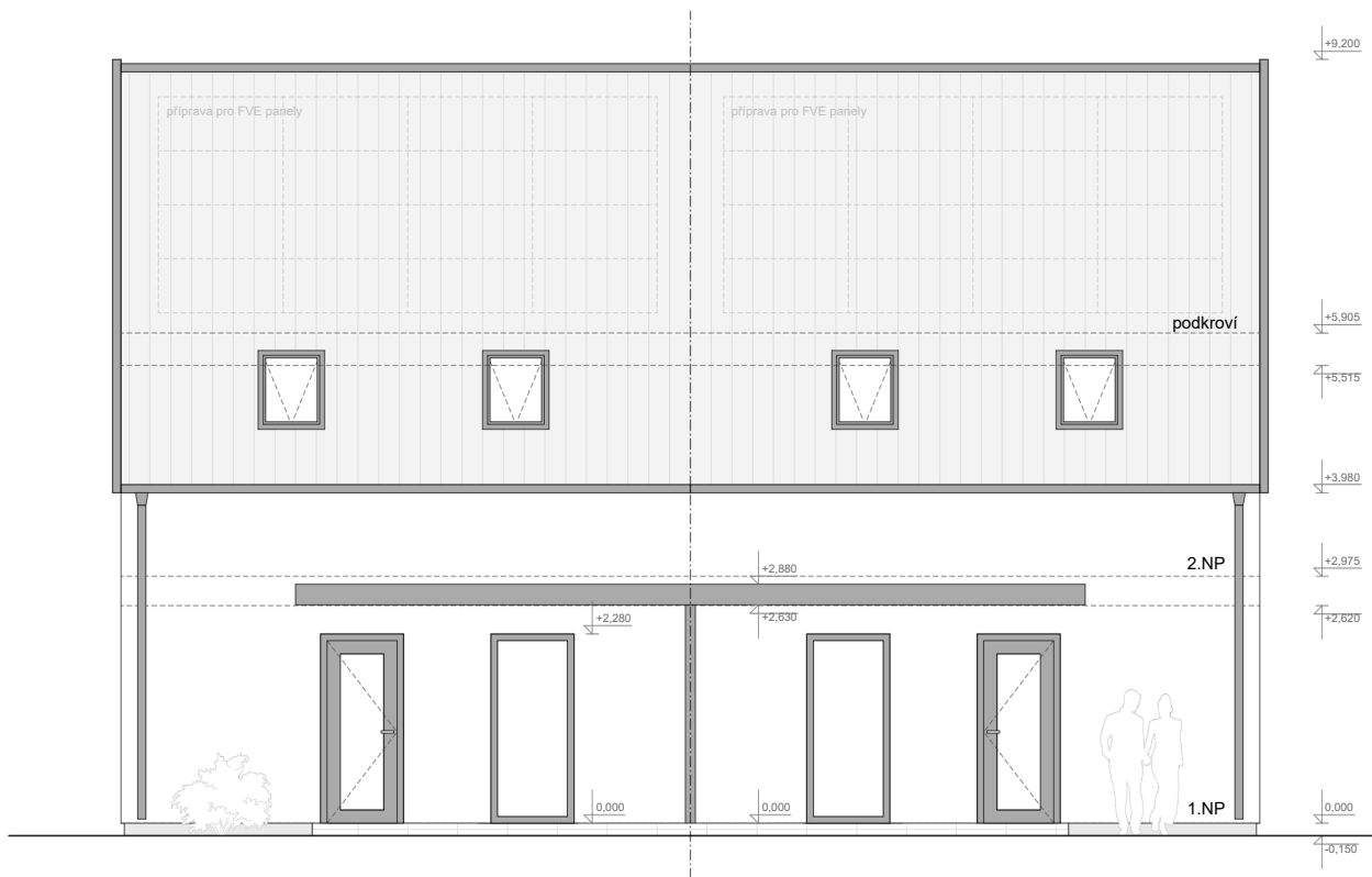
POHLED.Z ULICE
